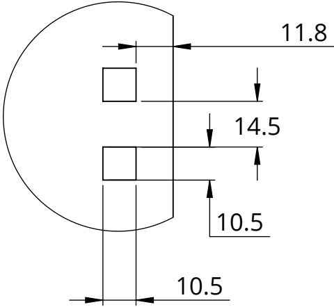
DÉTAIL A
